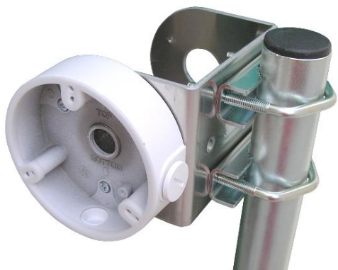
DH-PFA136 + DAH100L + 2x VBZ3 TWIN
